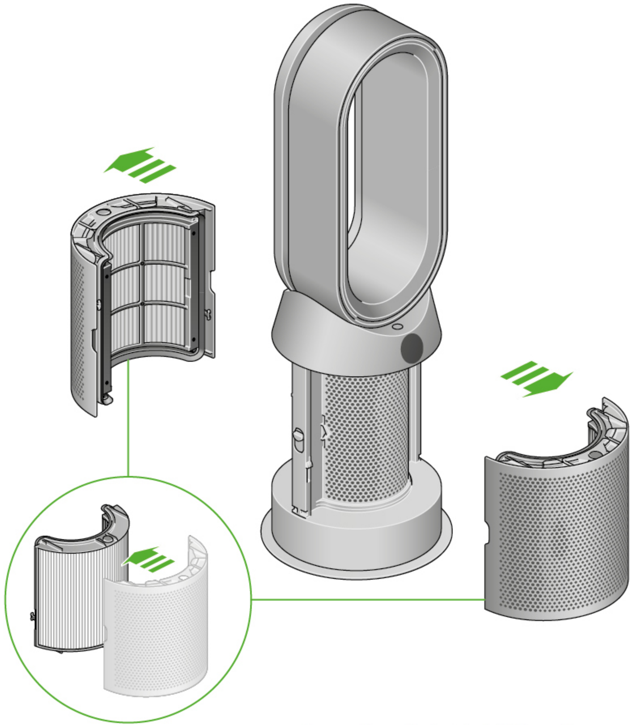
三合一暖風空氣清新機圖像，顯示濾網外殼打開，並展示出位於濾網外殼內的二合一 HEPA+ 活性炭濾網。箭咀指示濾網外殼需要安裝至產品底座之上。
